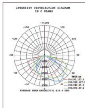
54W
