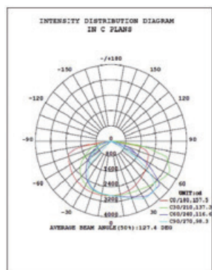
95W
